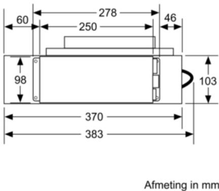
Aanzicht luchtuitlaat
