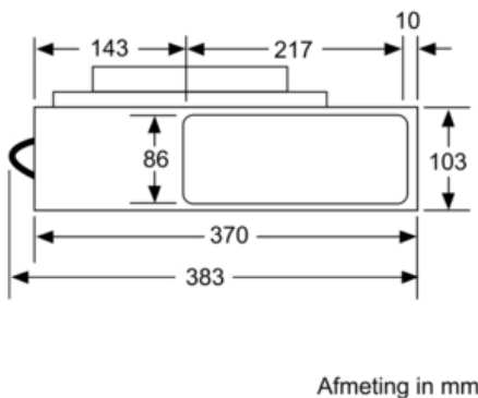
Aanzicht luchtuitlaat
