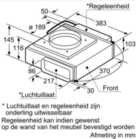
Aanzicht regeleenheid
