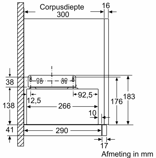
Positie LED lampen X: al naar gelang uitrusting Achterwandpaneel max. 20 mm Afmeting in mm
