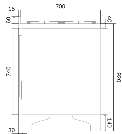
Zijaanzicht
