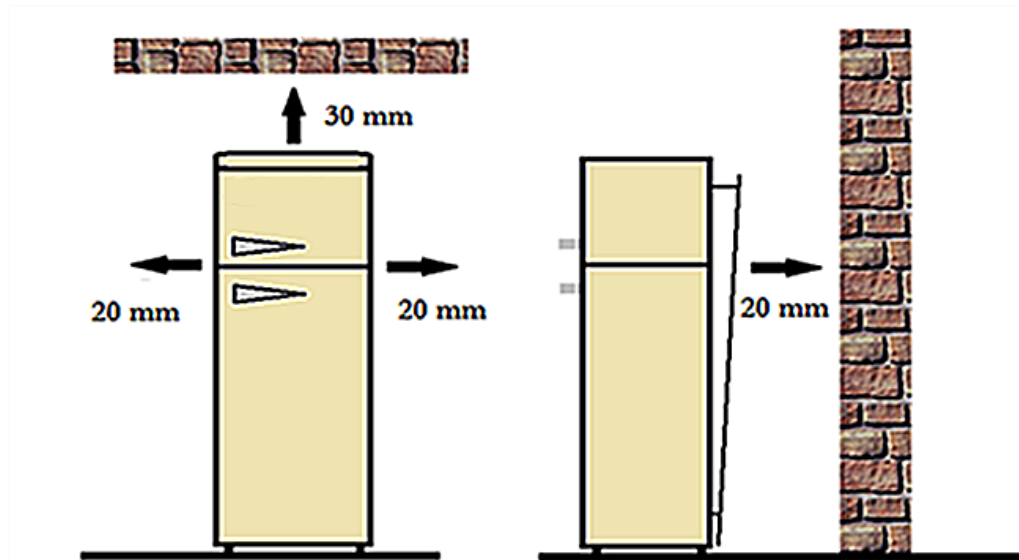
Mindestabstände
