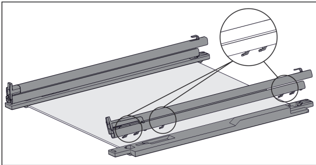
Fig. 42 Glasplaat met rails en vasthouddelen
