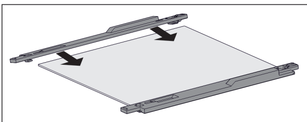
Fig. 44 Glasplaat met vasthouddelen
