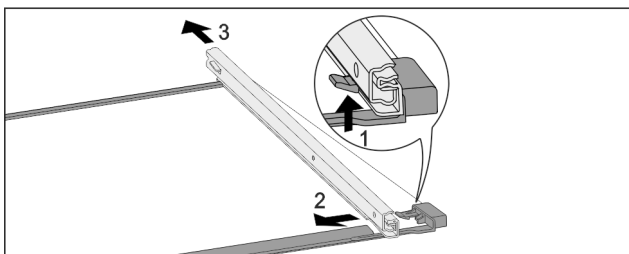
Fig. 37 Glasplaat met rails
