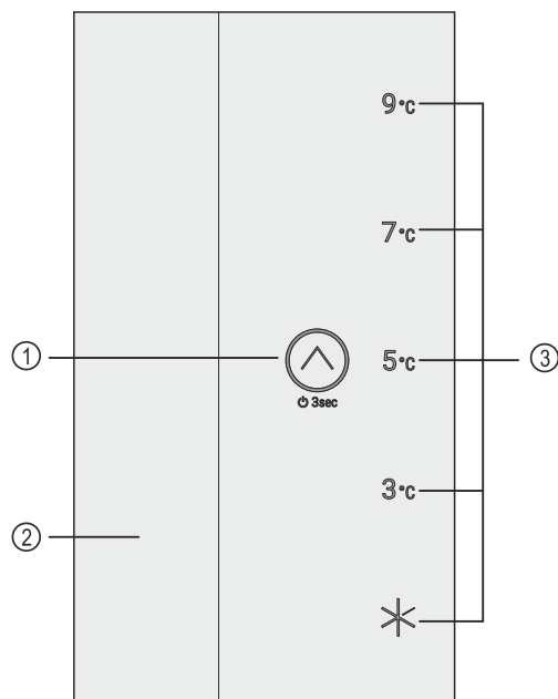
Fig. 26 Bedienings- en weergave-elementen
