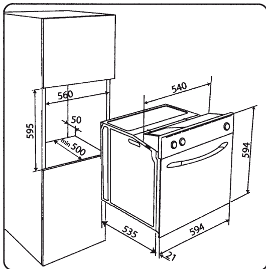
Fig. 2: Afmetingen BPM-60 en BPMD-60
